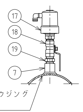
空気弁取付図 S=1:10
