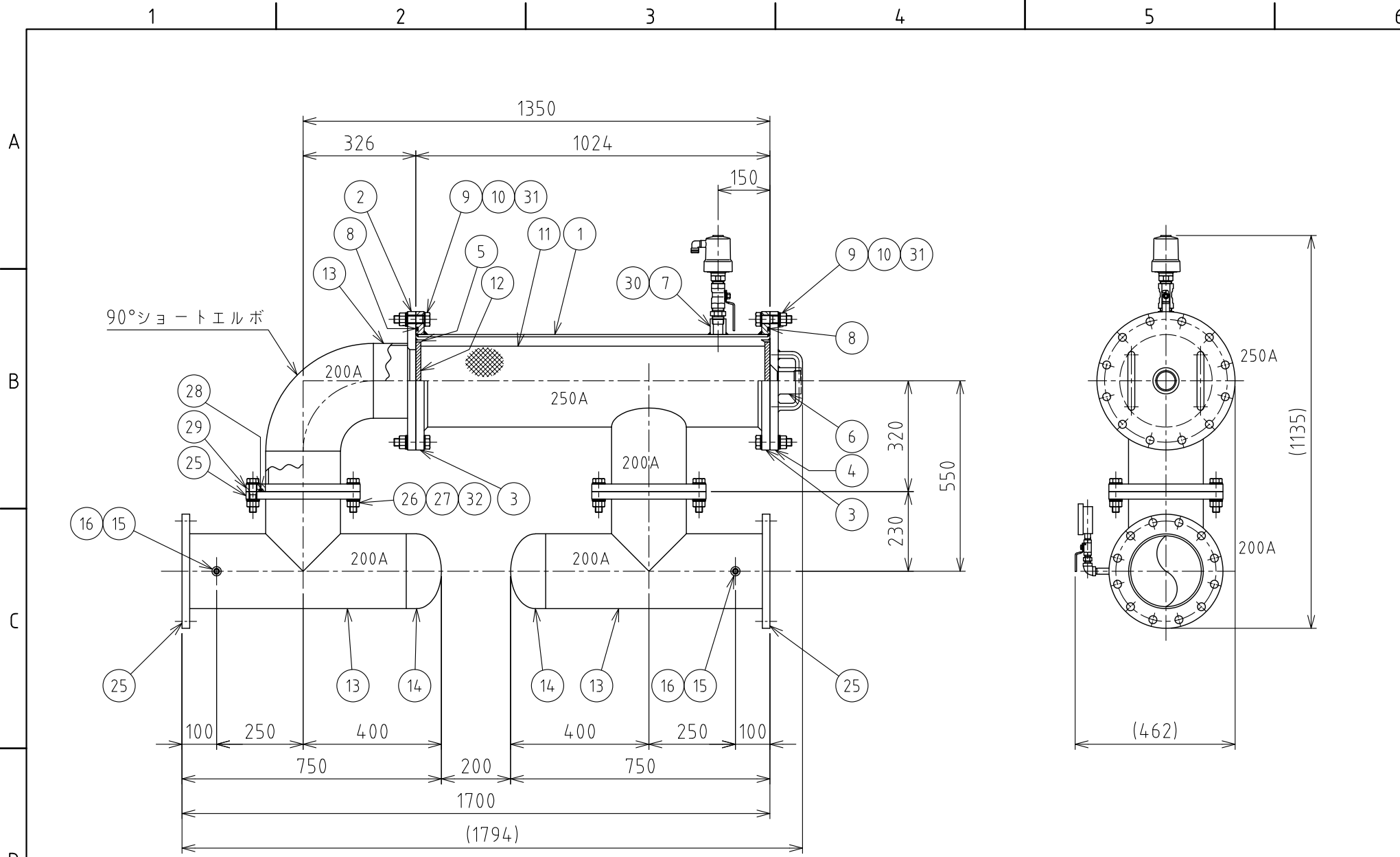
圧力計取付図 S=1:10
