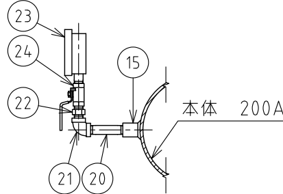
圧力計取付図 S=1:10
