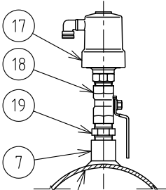
空気弁取付図 S=1:10
