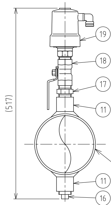
空気弁取付図 A 矢 視
