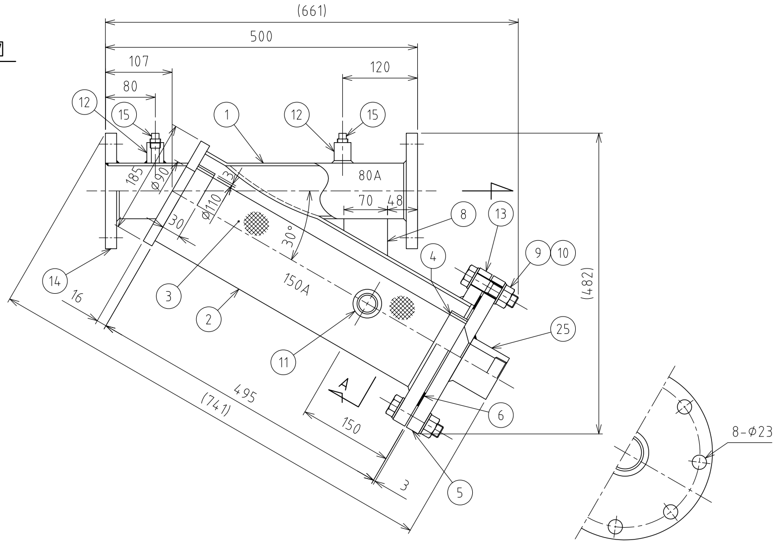
空気弁取付図 A 矢 視
