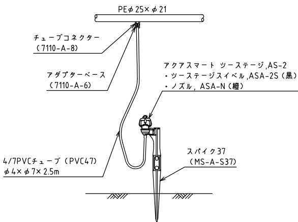
スピリクラー詳細図
