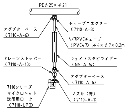
スプリンクラー詳細図
