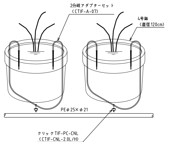
点滴かん水詳細図
