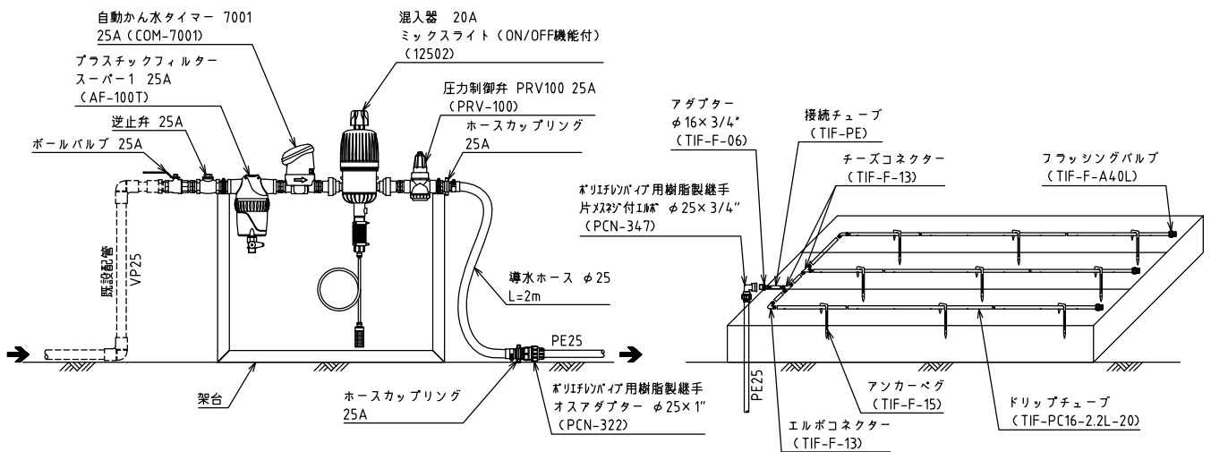
コントロールヘッド詳細図
