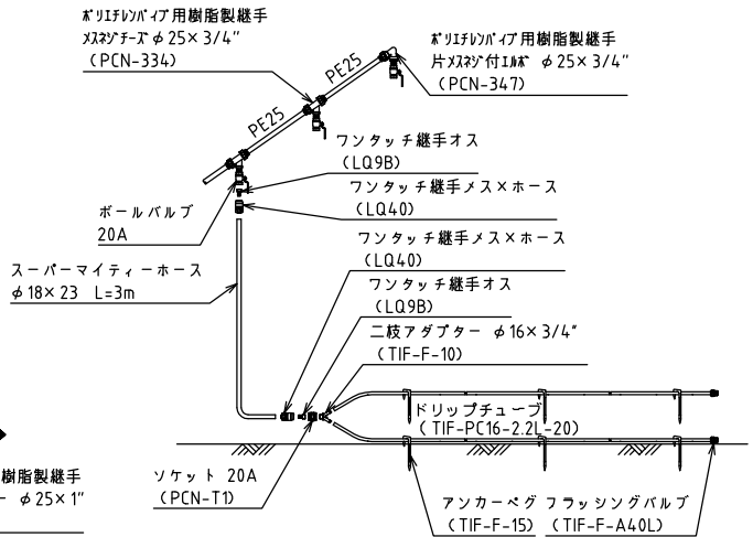
点滴かん水詳細図
